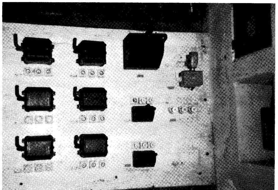
Die instandgesetzte Schalttafel in der Sakristei
